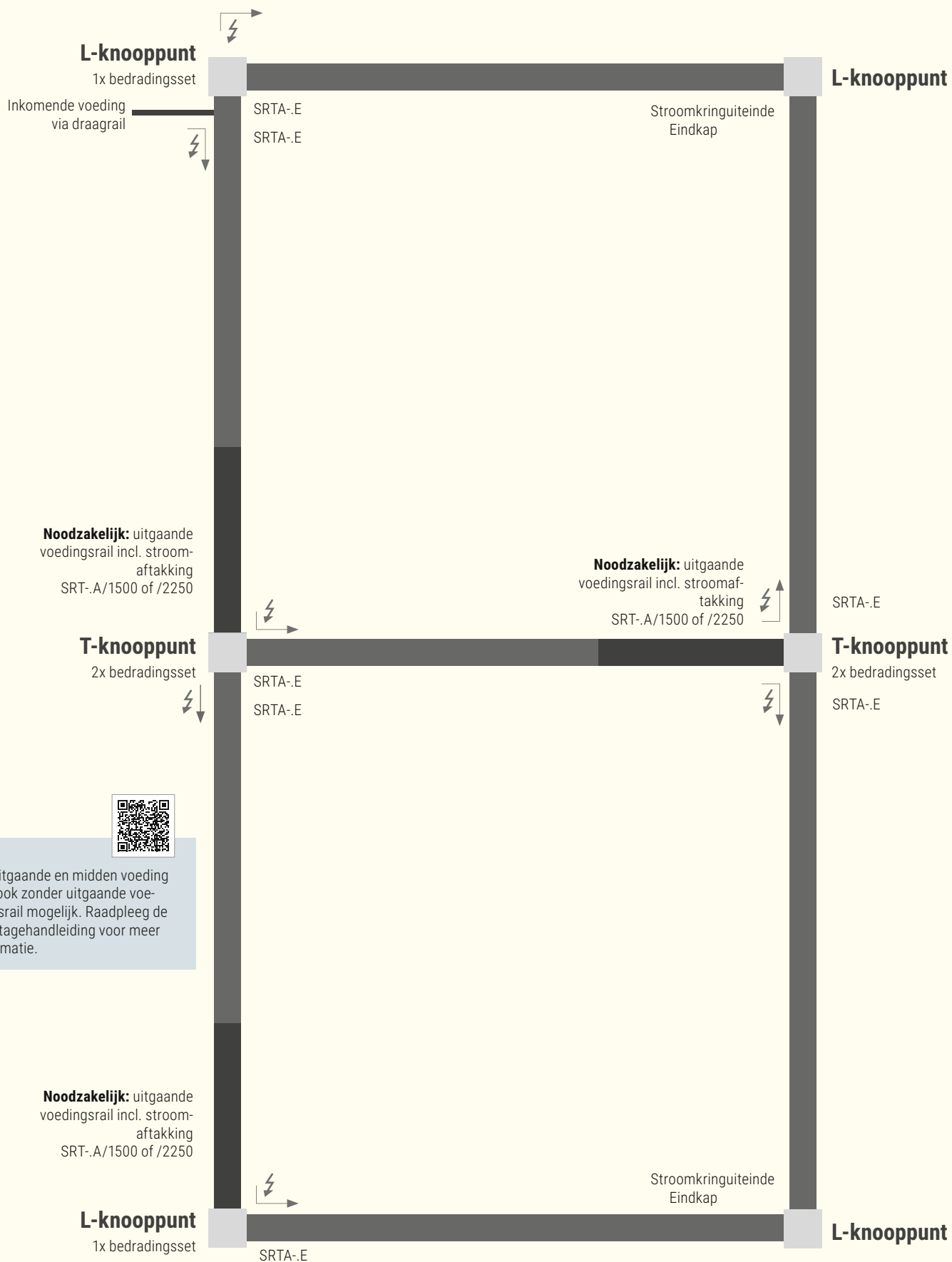
L-knooppunt SRT-KL
