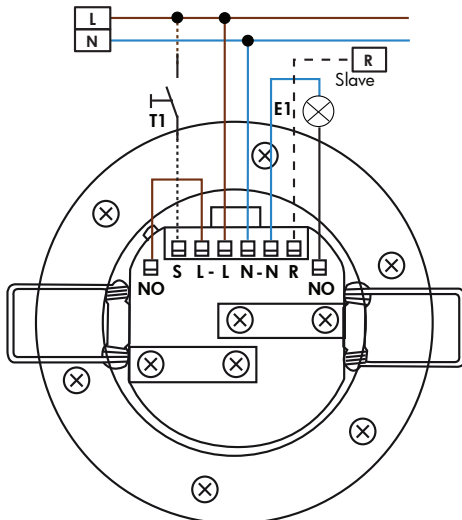
Schaltbild PD4-M-1C-DE
